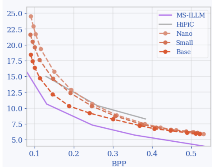
Tecnick Compression (FID)
